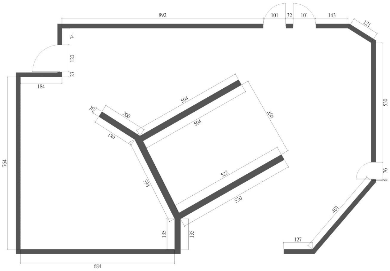
5F平面配置圖
